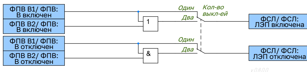
Рисунок 1.60 – Функциональная схема логики ФСЛ
