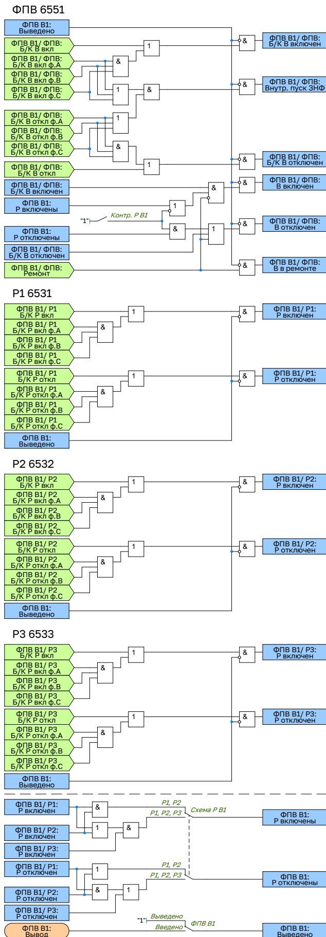
Рисунок 1.57 – Функциональная схема логики ФПВ В1
