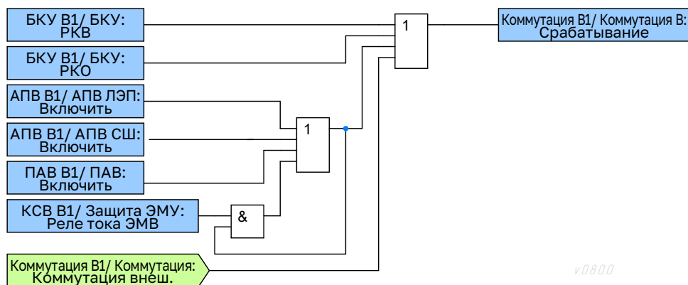
Рисунок 1.59 – Функциональная схема логики коммутации В1
