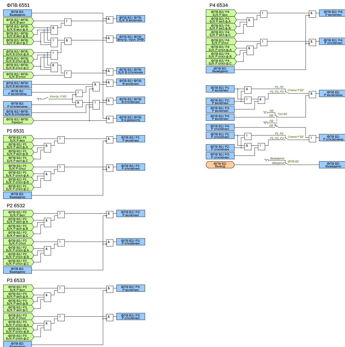
Рисунок 1.58 – Функциональная схема логики ФПВ В2
