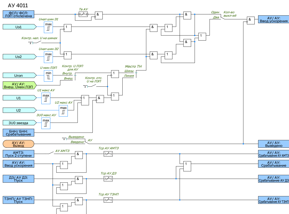
Рисунок 1.36 – Функциональная схема АУ
